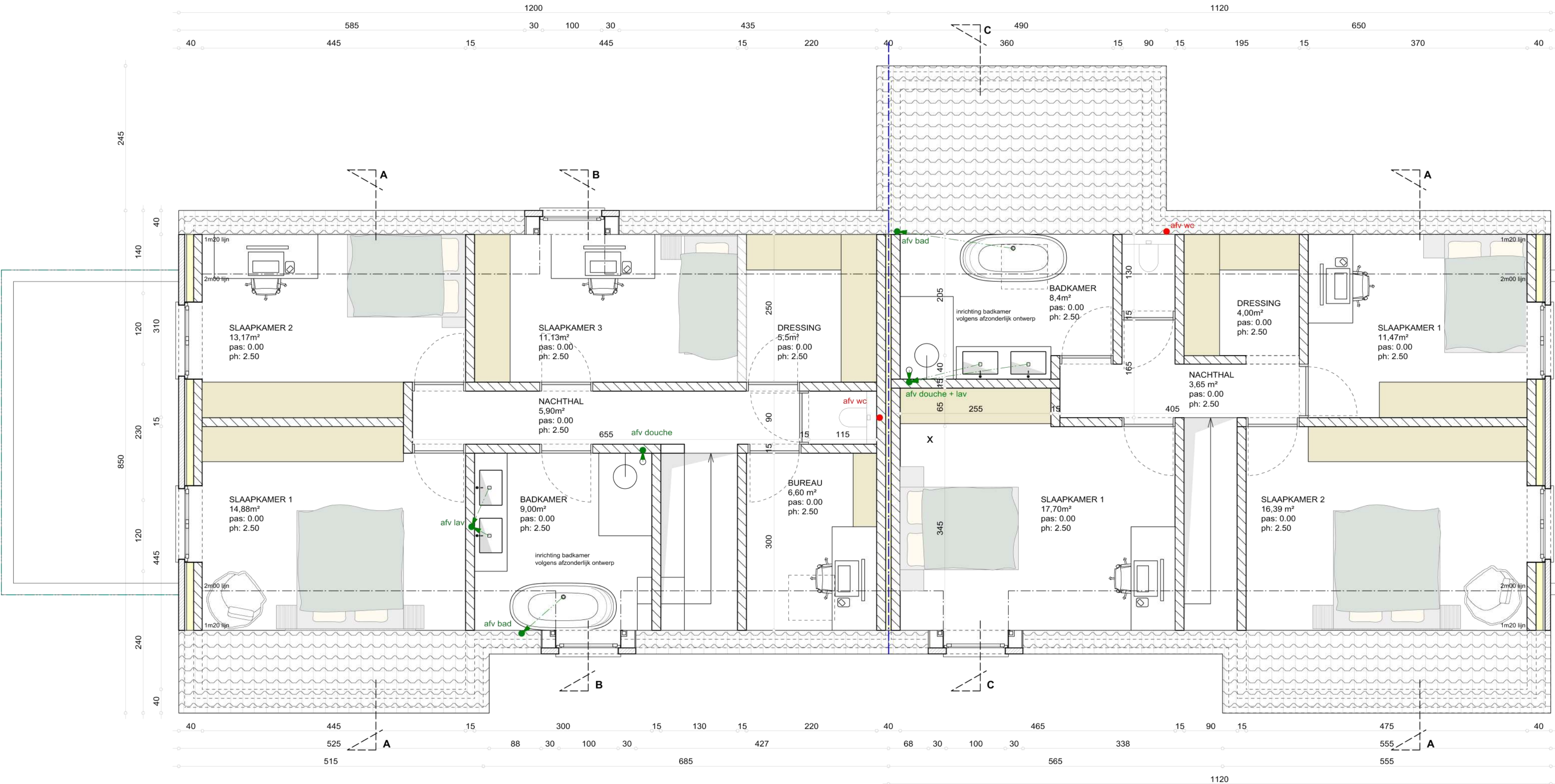
VERDIEPING nieuwe toestand 1/100
