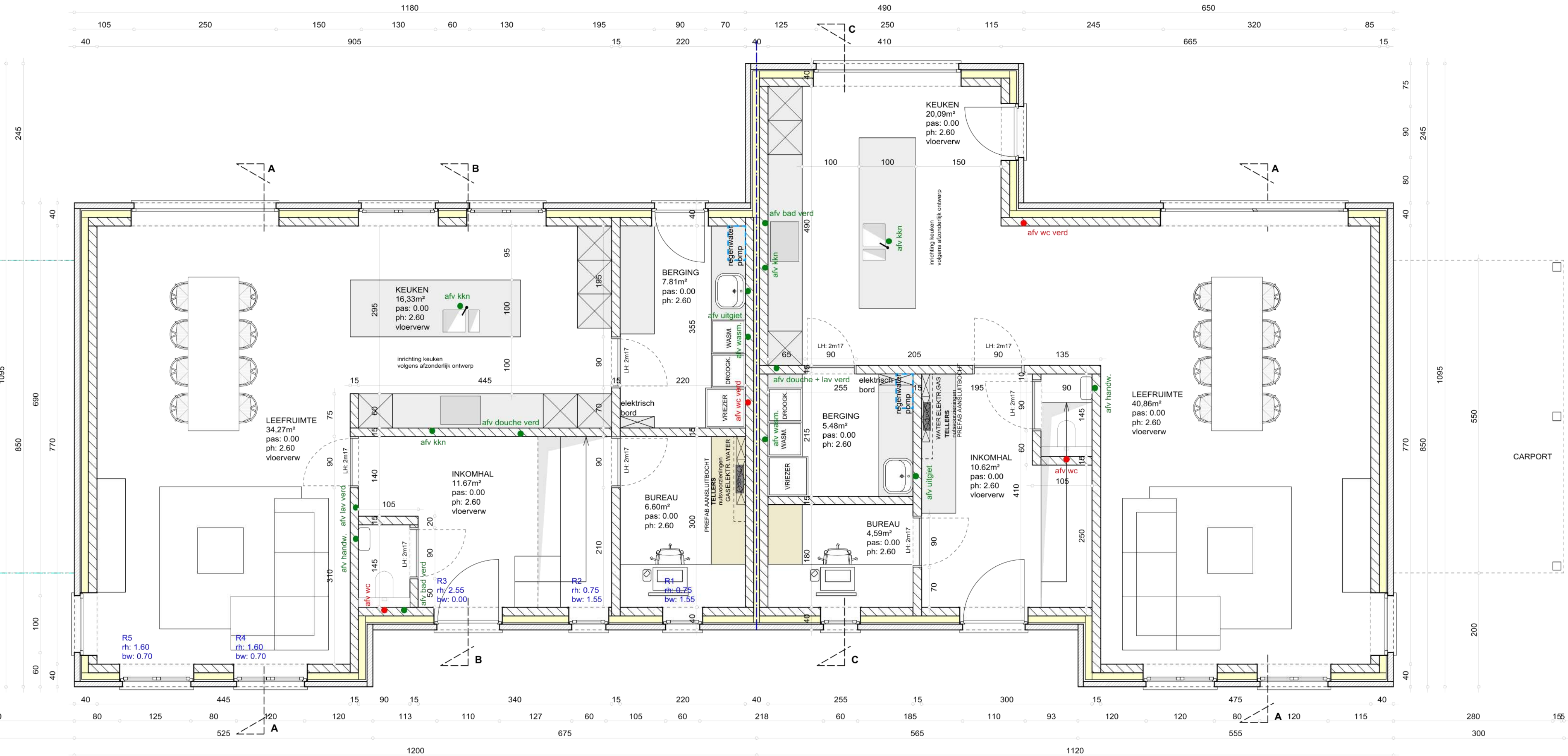
GELIJKVLOERS nieuwe toestand 1/50
